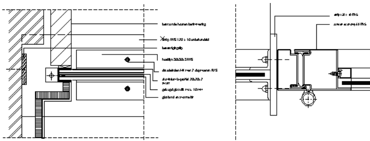
PRINCIPEDETAIL HORIZONTALE DOORSNEDE SCHAAL 1: 2
